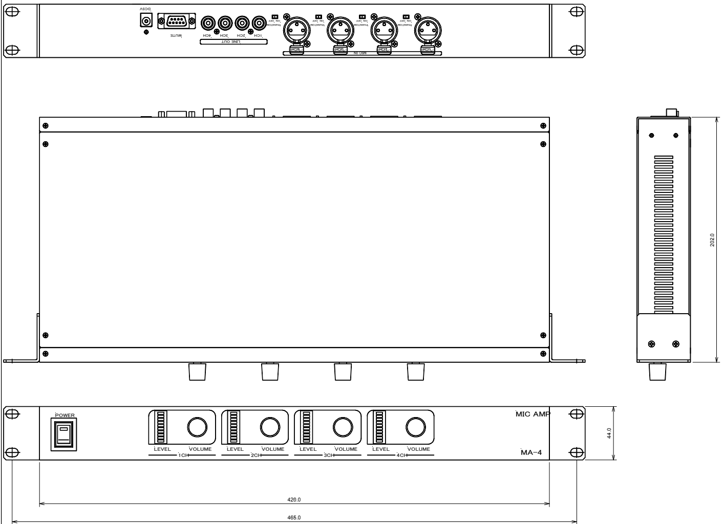
外形図
